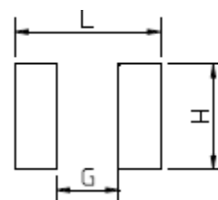
Land Pattern (Unit:mm)
