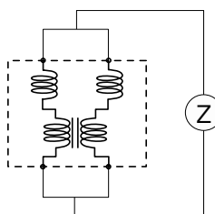
(B)共模
