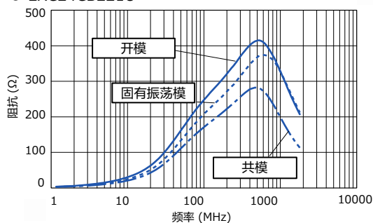
(A)开模
