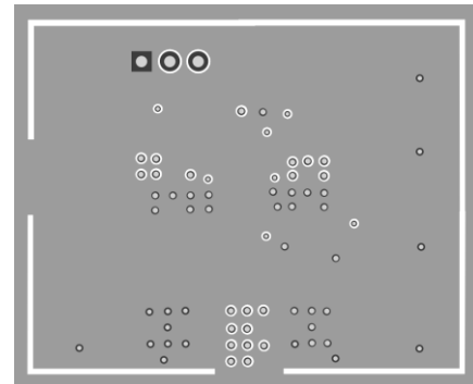
Inner Layer 1
