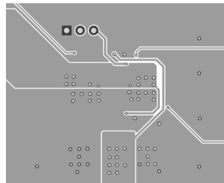
Inner Layer 2
