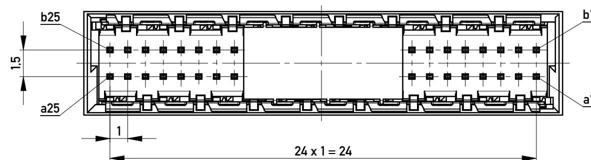
Leiterplatten-Layout Vorschlag / PCB-layout proposal
