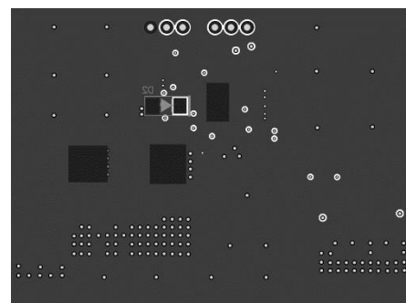
Bottom Layer
