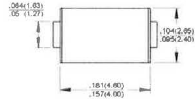
DO-214AC (SMA)
