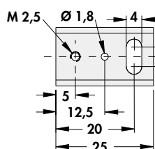
UK 14 SA 220
