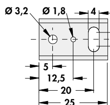
UK 14 SA 220 3.2
