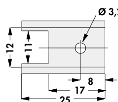
SK 431-2
