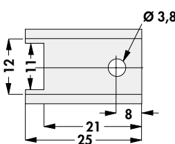
SK 431-1
