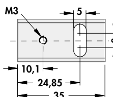
SK 13 35 SA 220
