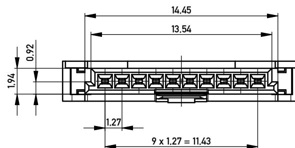
Einzelheit X - detail X M 2:1
