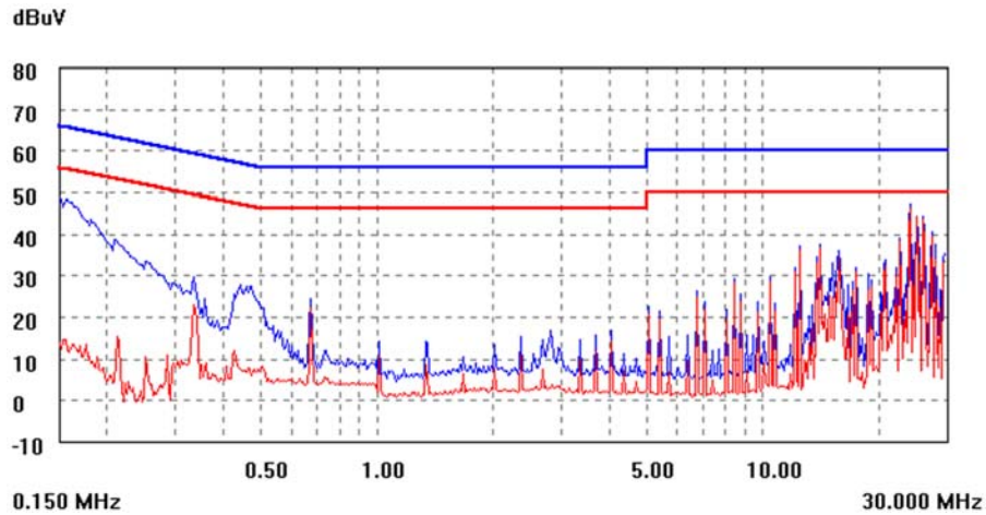
VIN = 48V, Io = Io,max, L Line
