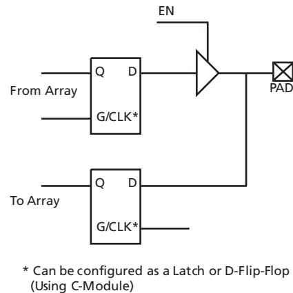
Figure 1-4 • I/O Module
