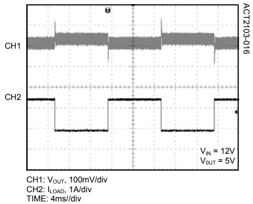
Load Transient (1.5A~3A)
