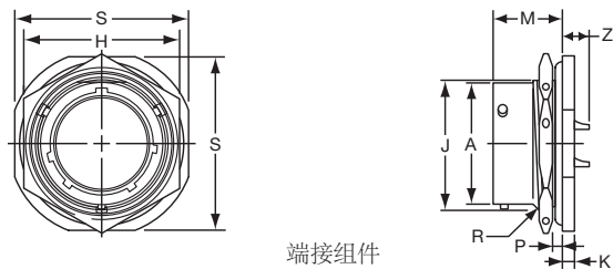
端接组件
