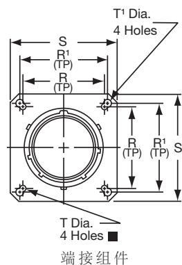
端接组件
