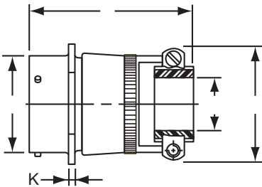
端接组件
