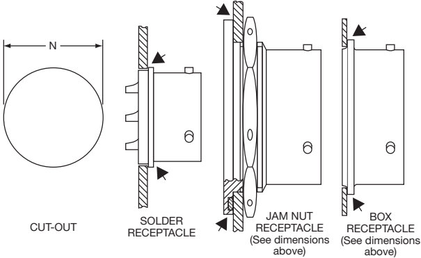
HERMETIC RECEPTACLES
