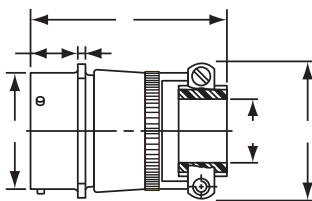
端接组件 “SE” (SR), MS / “F” 抗拉力电缆夹
