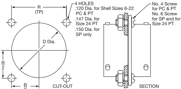
法兰盘安装连接器 FLANGE MOUNTED CONNECTORS
