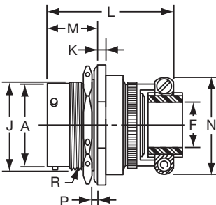
端接组件
