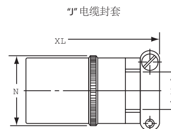
MS3110J-XX-XXX
