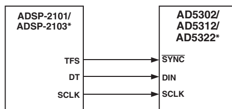
Figure 10. AD5302/AD5312/AD5322 to ADSP-2101/ADSP-2103 Interface
