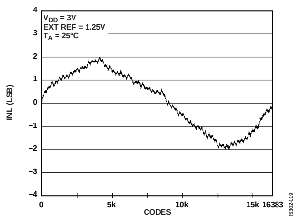
Figure 20. INL AD5648-1
