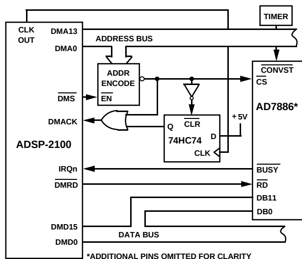
Figure 17. AD7886-ADSP-2100 Interface
