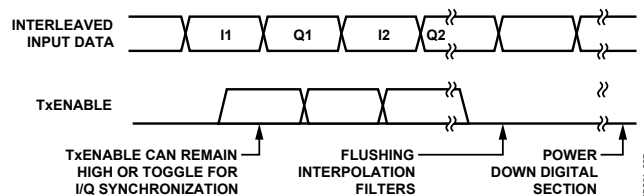
Figure 91. TXENABLE Function
