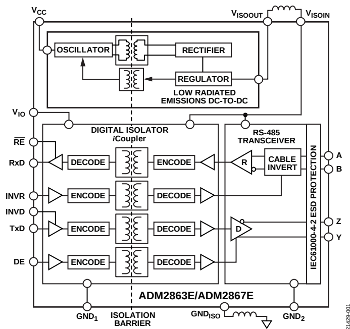
Figure 1. ADM2863E/ADM2867E
