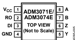
Figure 5. ADM3071E/ADM3074E Pin Configuration
