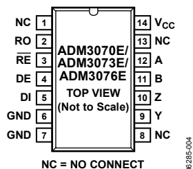
Figure 4. ADM3070E/ADM3073E/ADM3076E Pin Configuration
