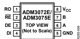
Figure 6. ADM3072E/ADM3075E Pin Configuration
