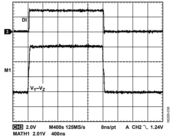
Figure 30. ADM3073E/ADM3074E/ADM3075E Driver Propagation Delay (500 kbps)
