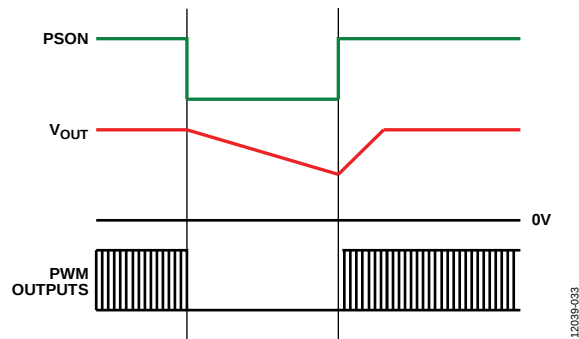
Figure 27. Prebias Startup
