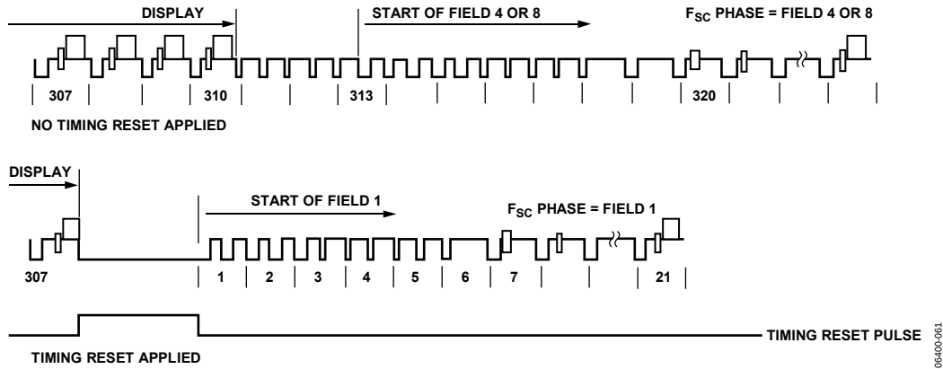
Figure 59. SD Timing Reset Timing Diagram (Subaddress 0x84, Bits[2:1] = 10)
