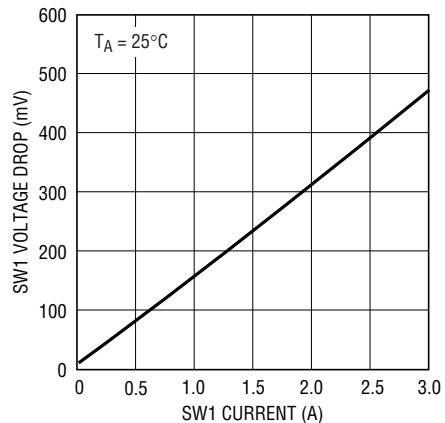
SW1 V_{\text{CESAT}}
