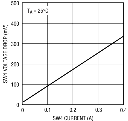
SW4 V_{\text{CESAT}}
