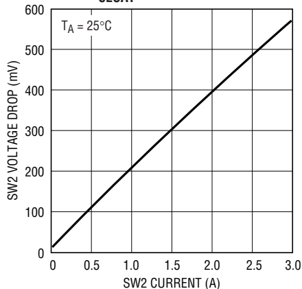
SW2 V_{\text{CESAT}}
