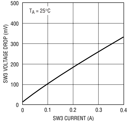
SW3 V_{\text{CESAT}}
