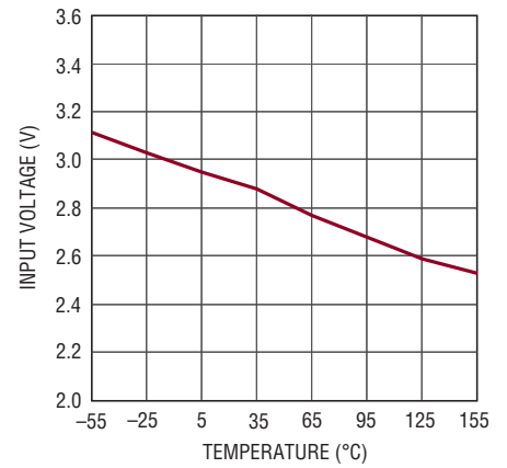
V_{IN} UVLO
