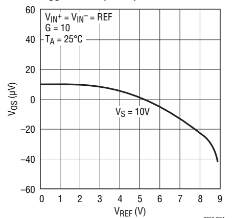
V_{OS} vs REF (Pin 5)
