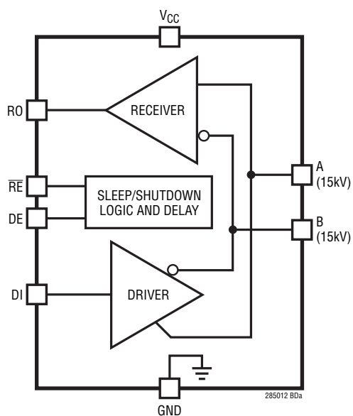
LTC2850
