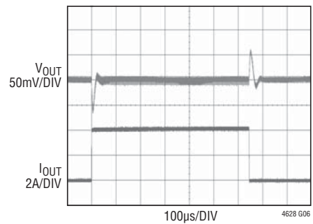
1.2V Load Transient
