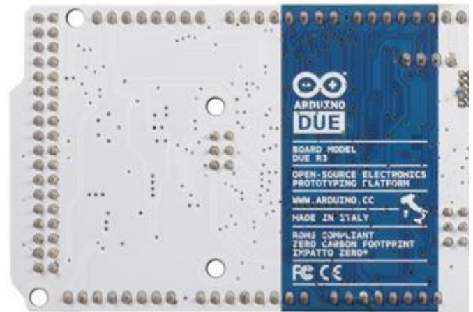
Arduino Due Back
