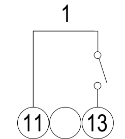
Fig. 6 Digital input 1
