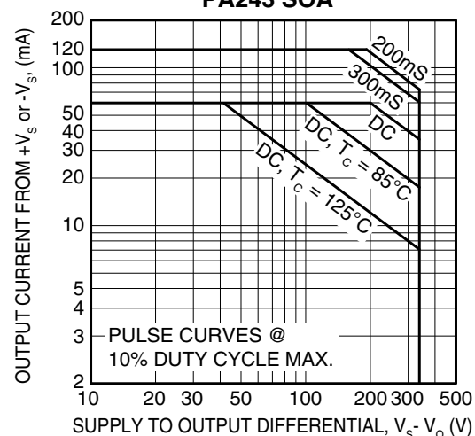
PA243 SOA
