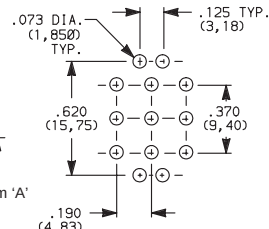
7301MD9_BE 3PDT
