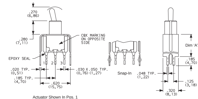
7101MD9__BE SPDT
