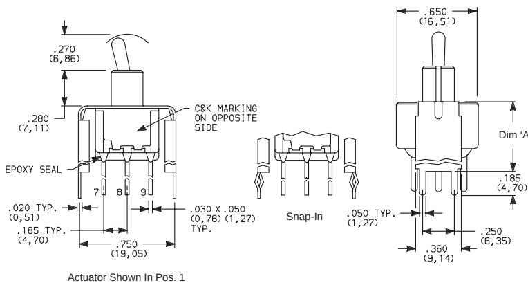
7301MD9__BE 3PDT
