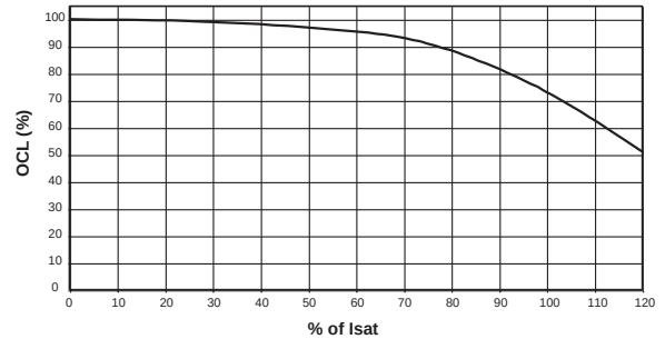
OCL vs Isat SDQ25
