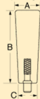
Projecting Stud
