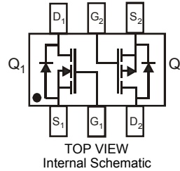
SOT-363
