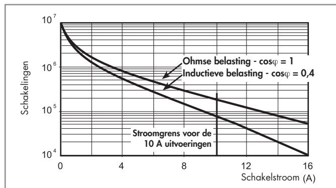
F 40 - Elektrische Levensduur bij AC Types 40.11/41
