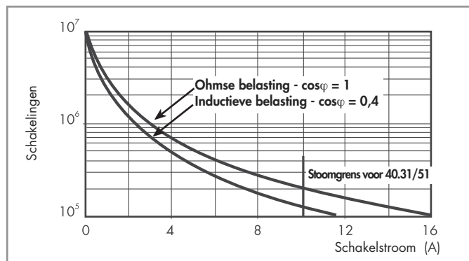
F 40 - Elektrische Levensduur bij AC Types 40.31/51/61
