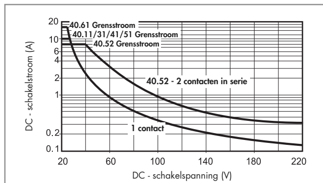
H 40 - Gelijkstroomvermogen bij DC1 belasting
