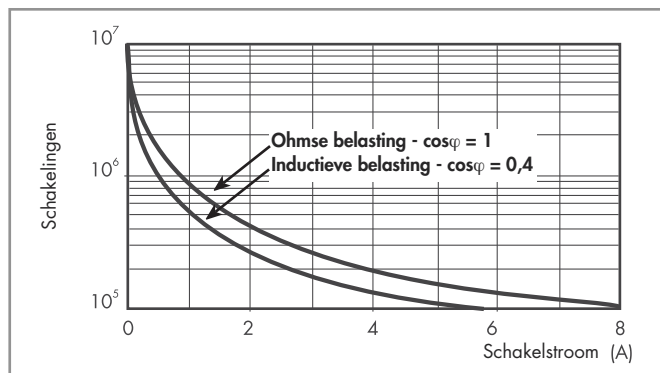
F 40 - Elektrische Levensduur bij AC Type 40.52
