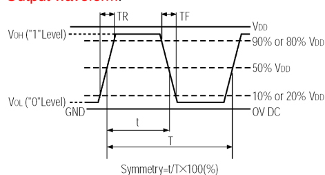
Output waveform:
