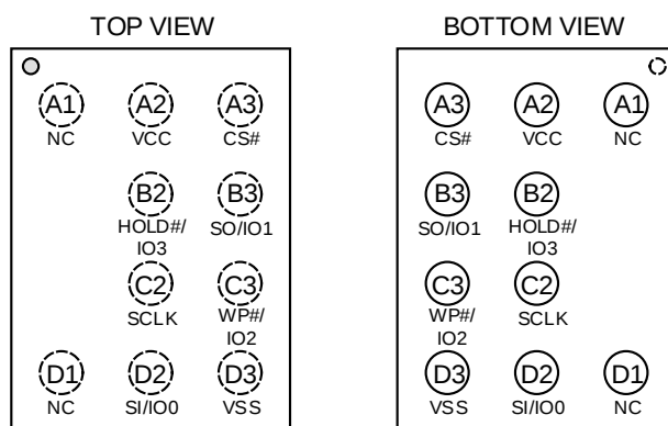
WLCSP
