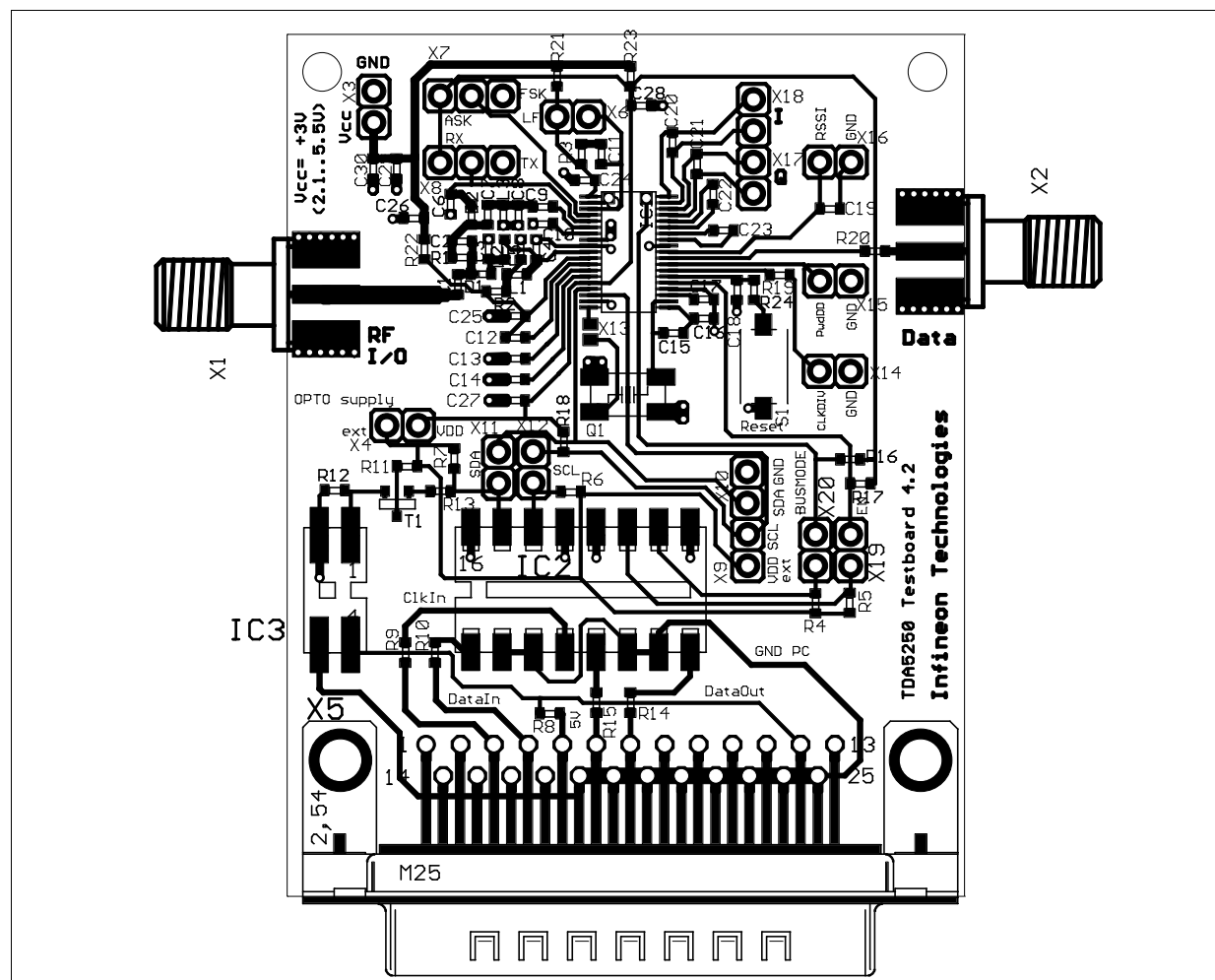
TDA5250 v42 layout.pdf
