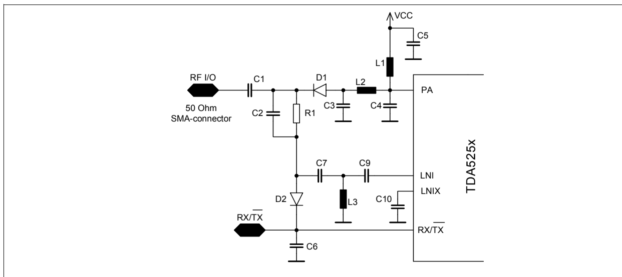
RX/TX_Switch.wmf
