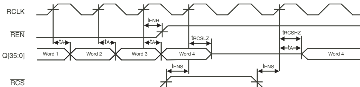
Figure 14. Output Enable
