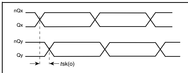
Output Skew
