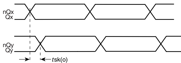
OUTPUT SKEW
