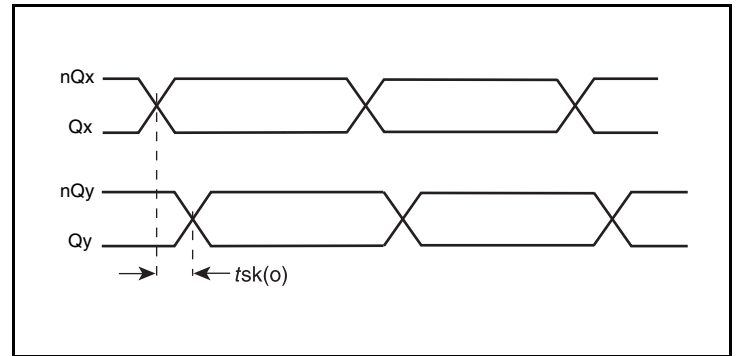
Output Skew
