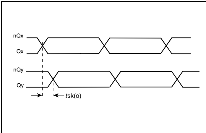
Output Skew
