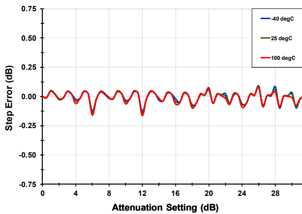
DNL [2800 MHz]
