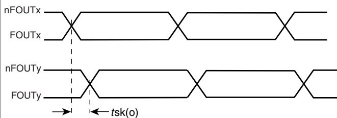
OUTPUT SKEW
