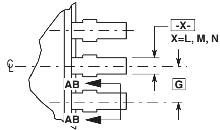
VIEW Y
