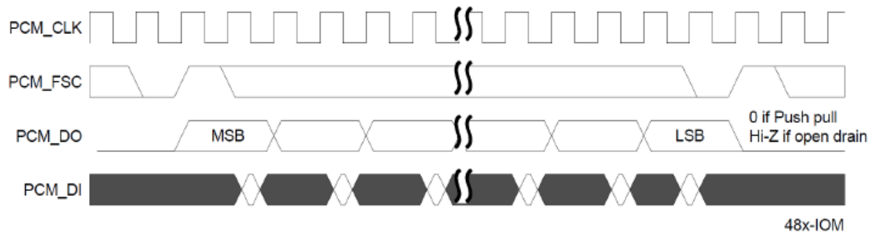
Figure 49 IOM format
