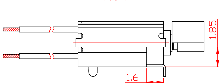
C 向视图
