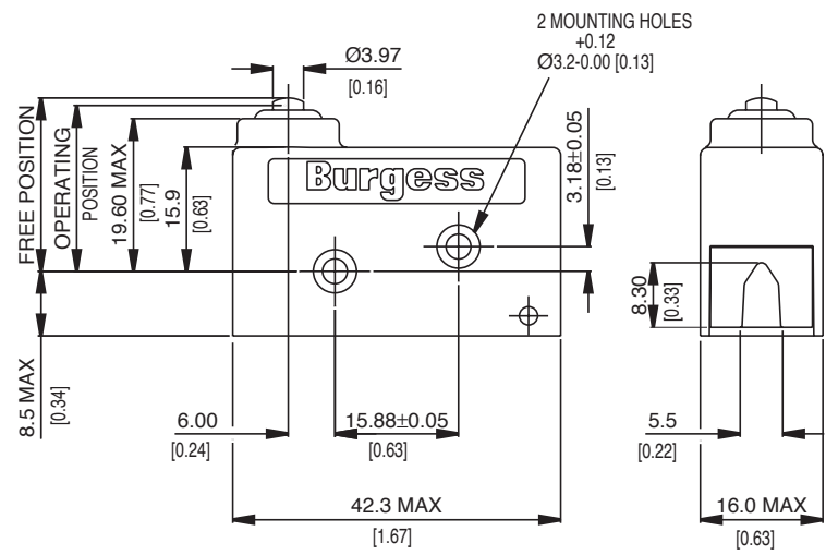
Dimensions
