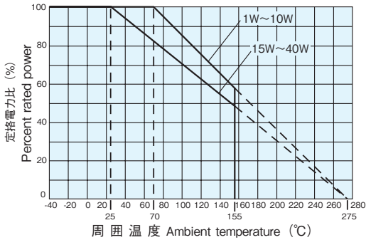
■負荷軽減曲線 Derating Curve
