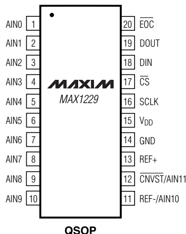
QSOP
