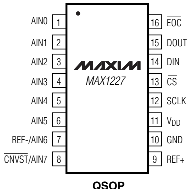
QSOP
